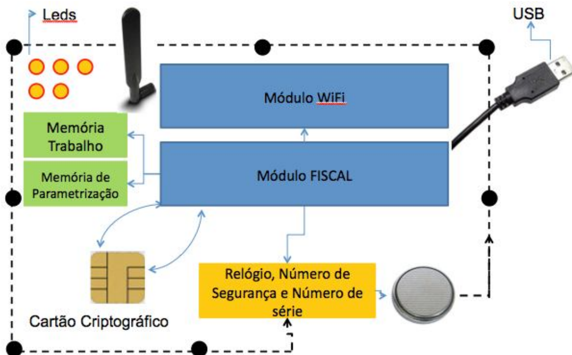
Figura 3 – Exemplo de implementação de um Equipamento SAT com interface de comunicação WiFi
